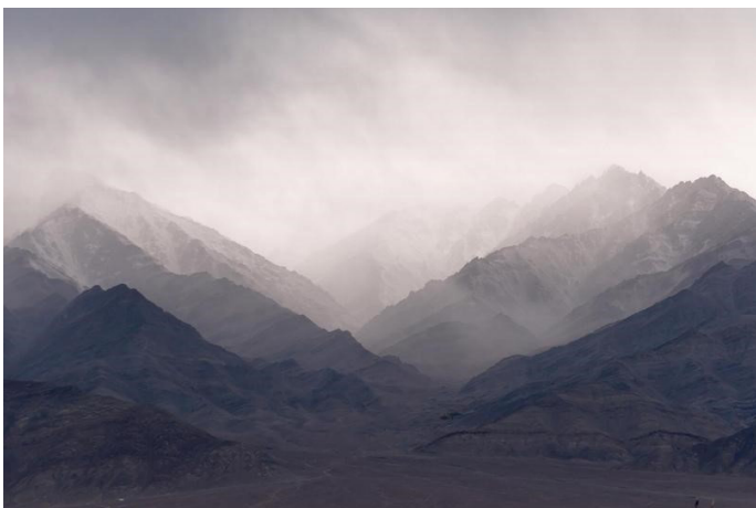
Воздушная перспектива
