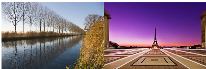
Линейная перспектива
