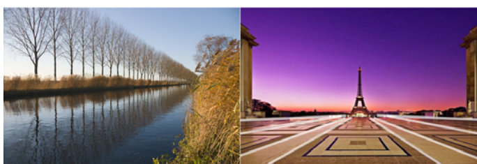
Линейная перспектива
